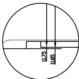
细节 I 比例 6:1
